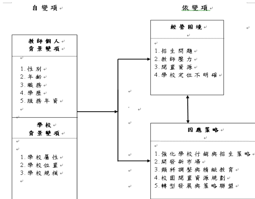
圖 1 研究架構圖
